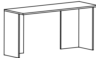
L.170 - P.58,6 - H.75,2
